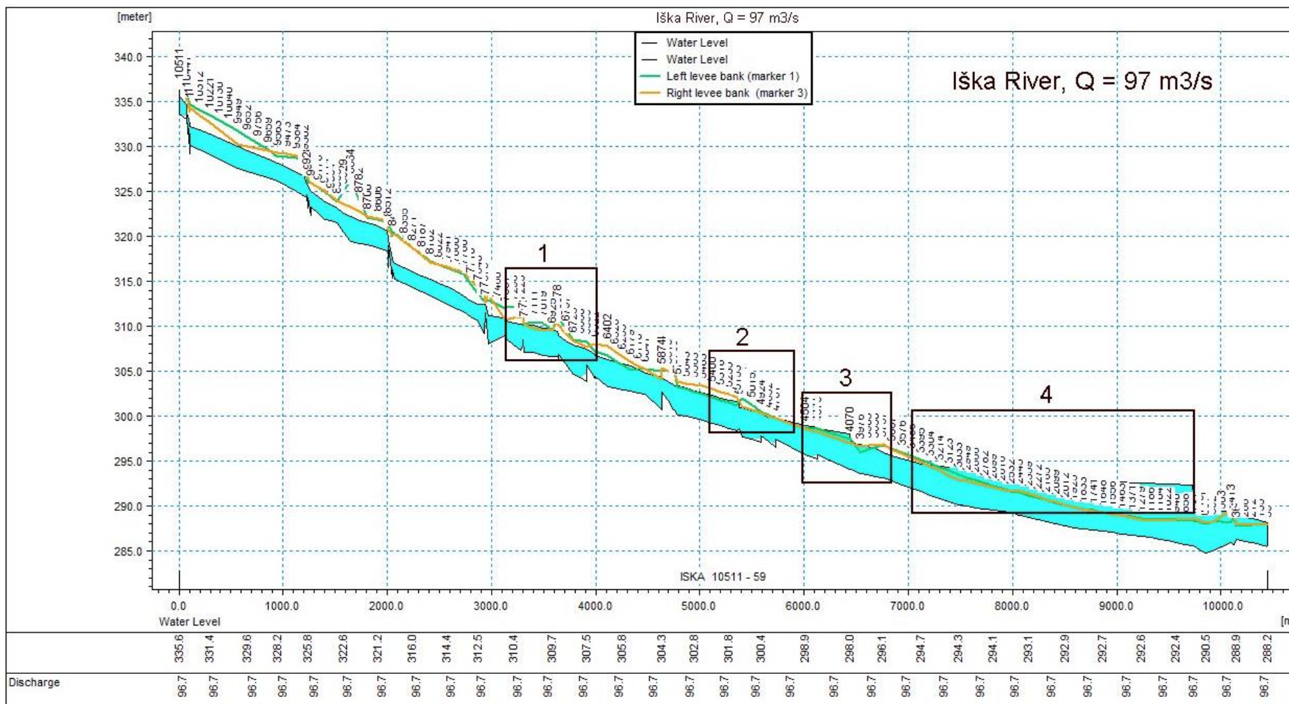
Slika 13: Vzdolžni profil reke Iške in kote vode pri pretoku 97 m 3 /s. Lokacije preliivanja se prikazuje na sliki 12
