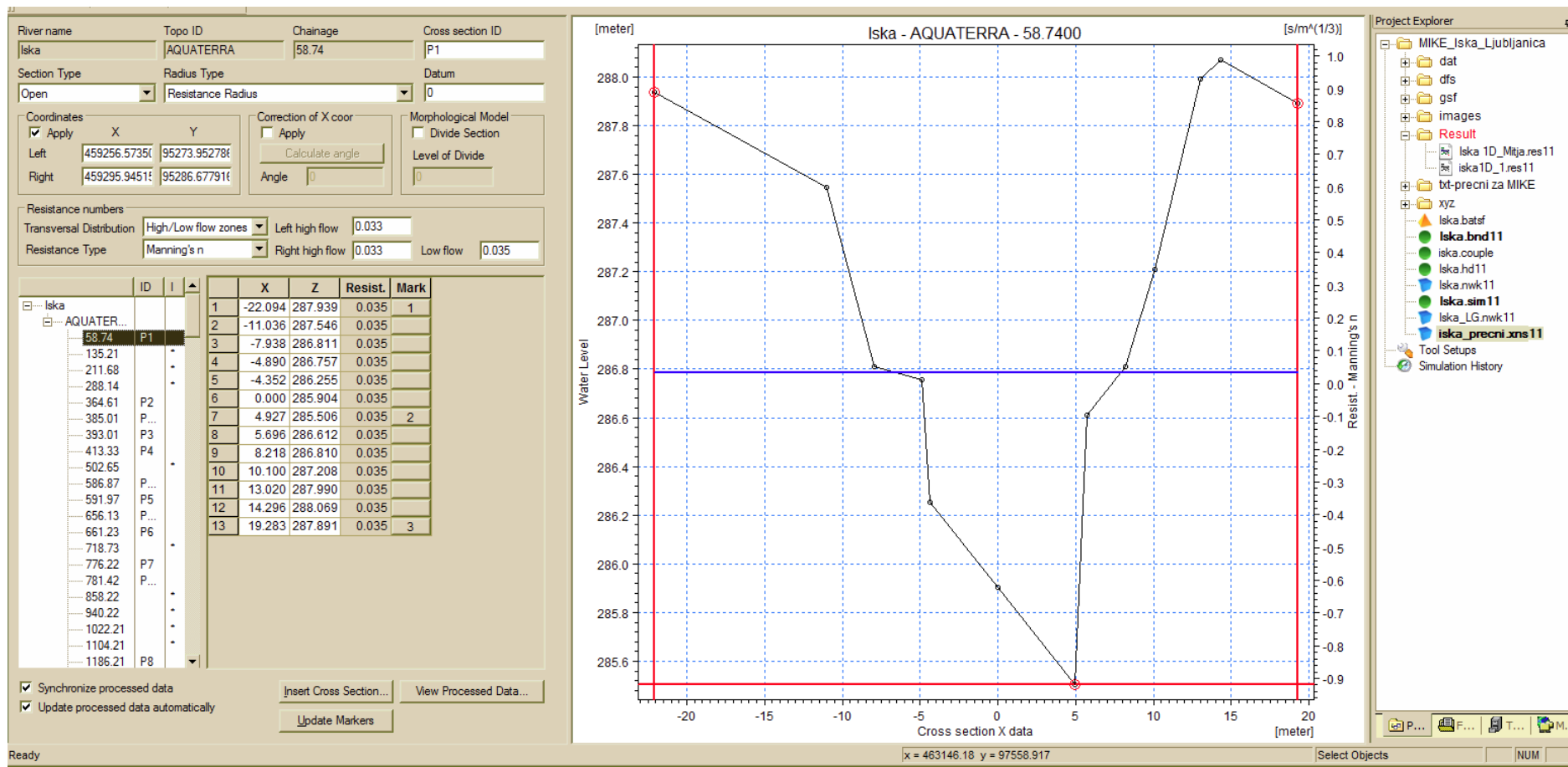
Slika 10: Slika profila št. 1 na Iški (prikaz profila 1 v programu MIKE 11)
