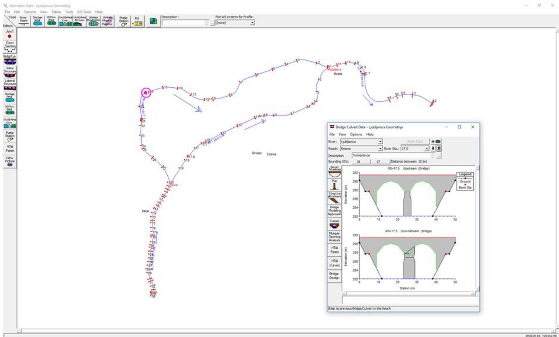
Slika 17: Situacija s prečnimi prerezi in prečni prerez pri Tromostovju.
