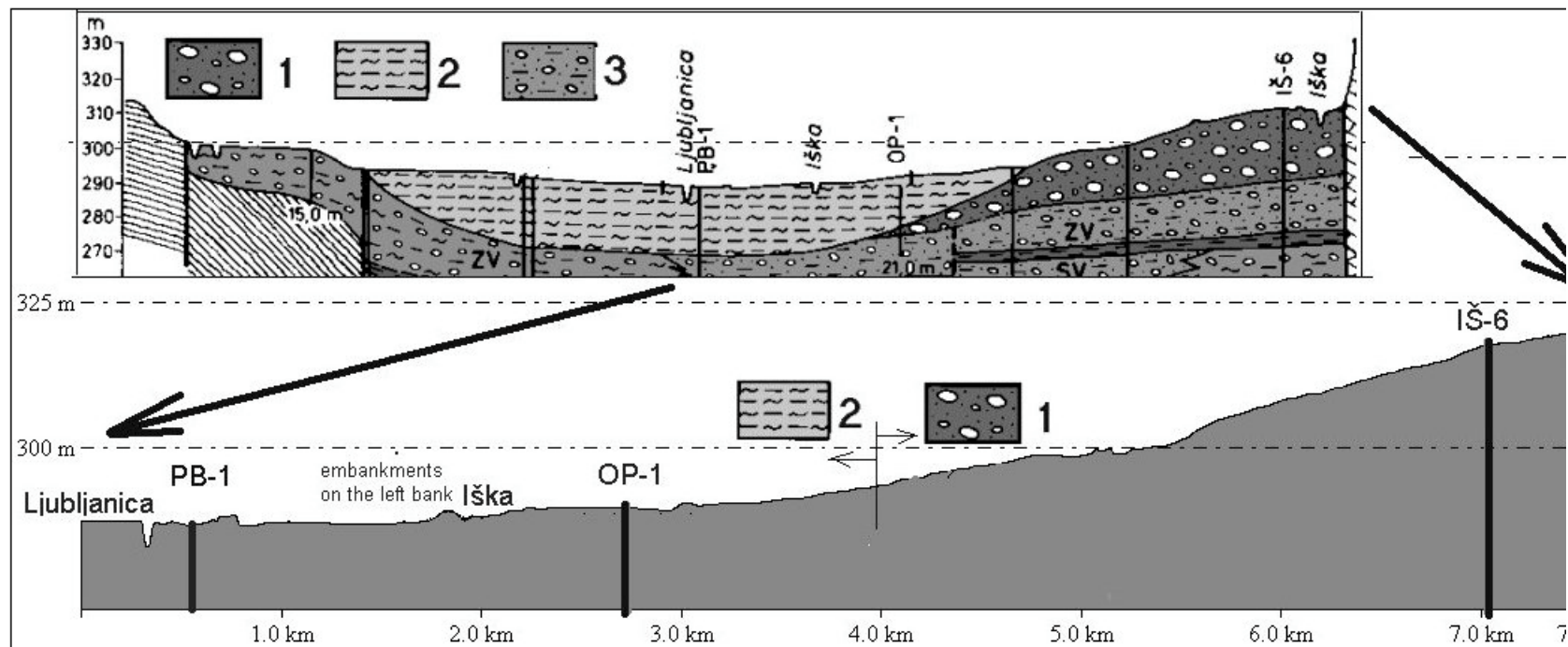
Slika 6: Hidrogeološki profil ob Iški (pozicija na sliki 4). Hidrogeološka enota št. 1 predstavlja prod s peskom in muljem v Iškem vršaju, št. 2
