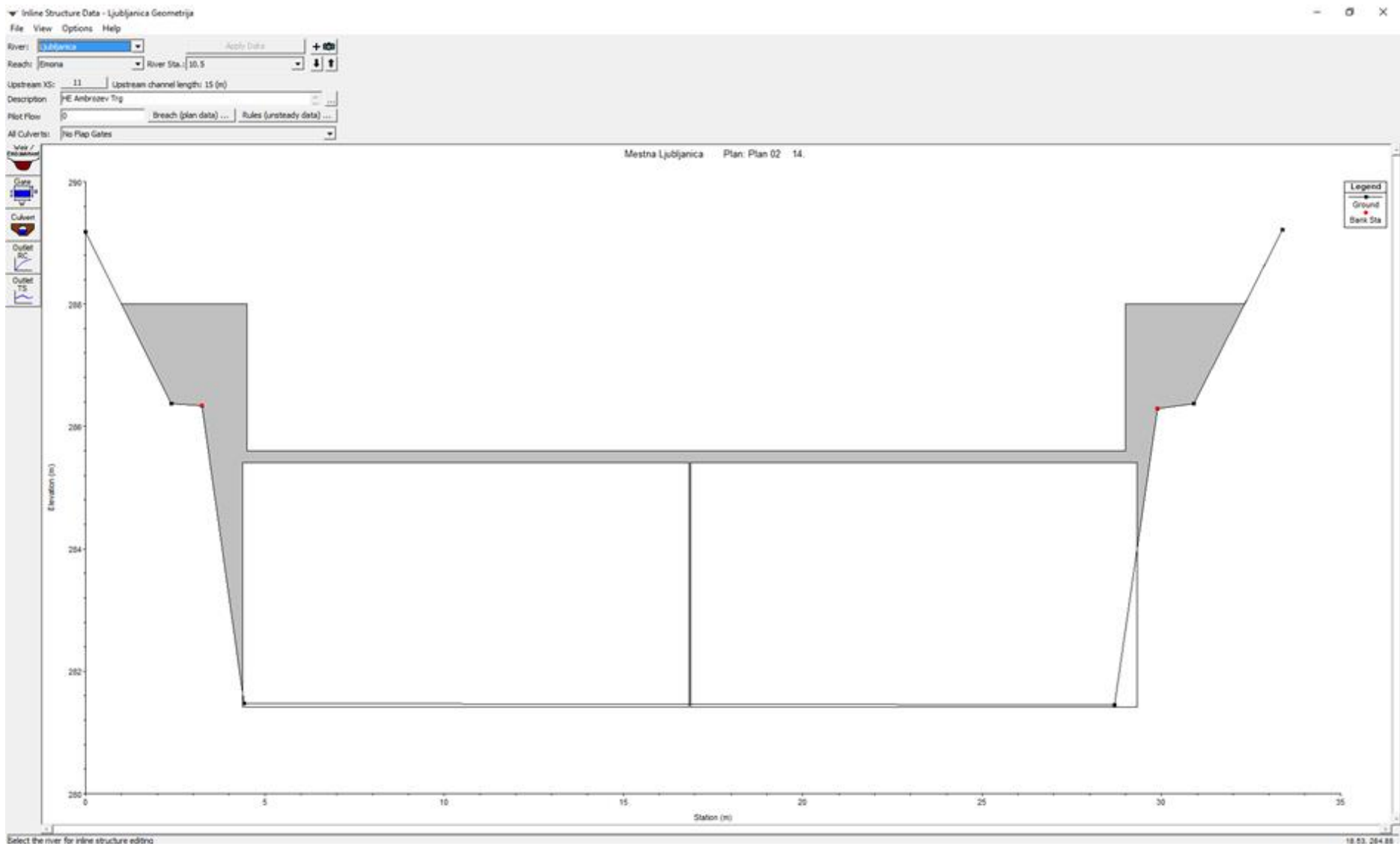
Slika 18: Prečni prerez pri zapornicah na Ambroževem trgu
