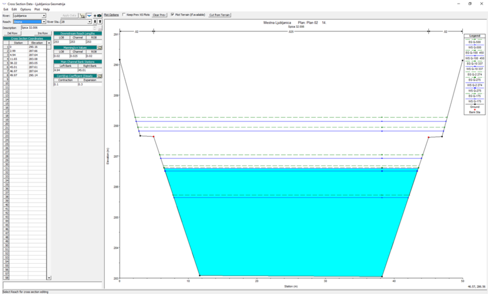
Slika 21: Prečni prerez Mestne Ljubljance
