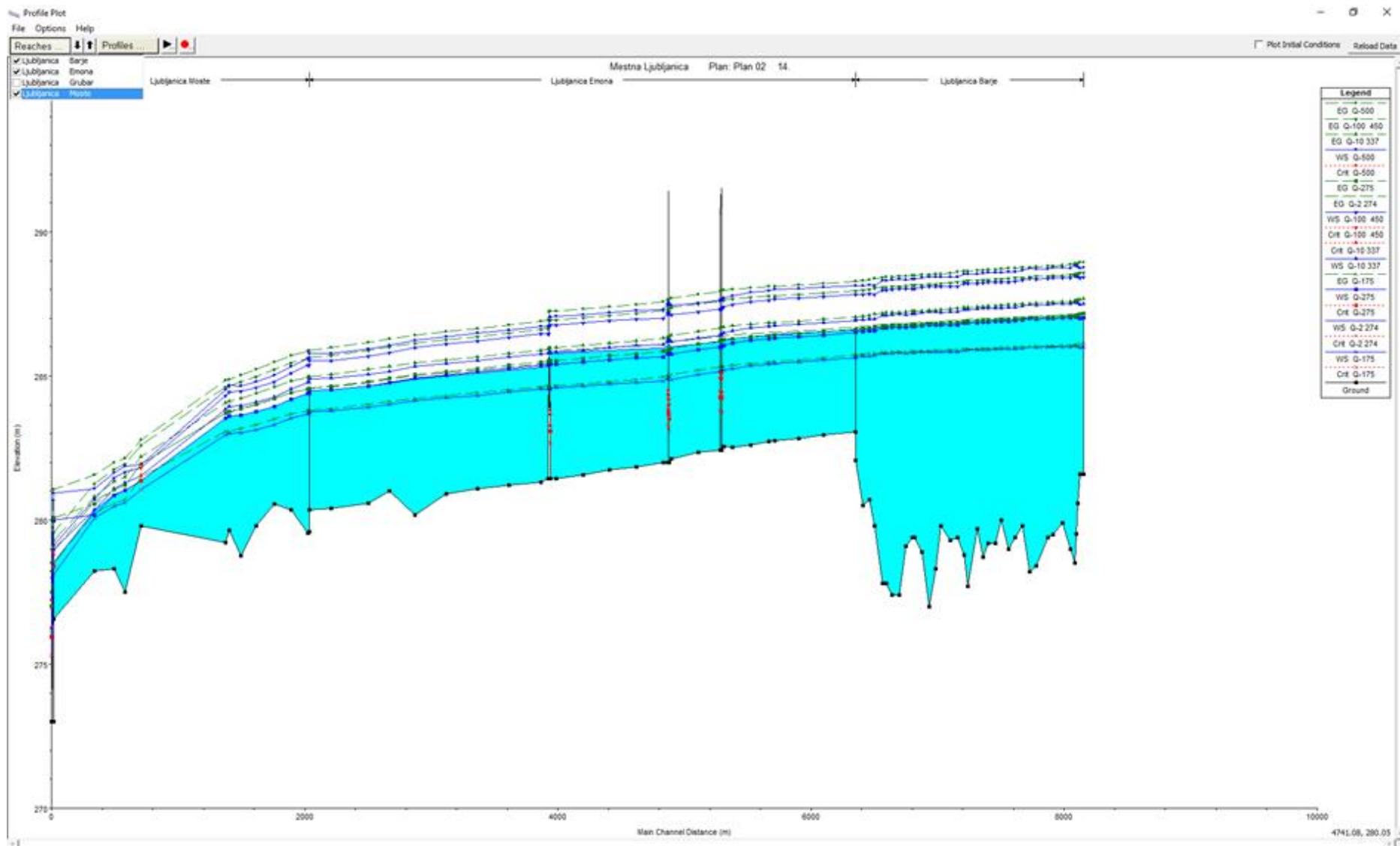
Slika 16: Vzdolžni prerez Barje-Moste
