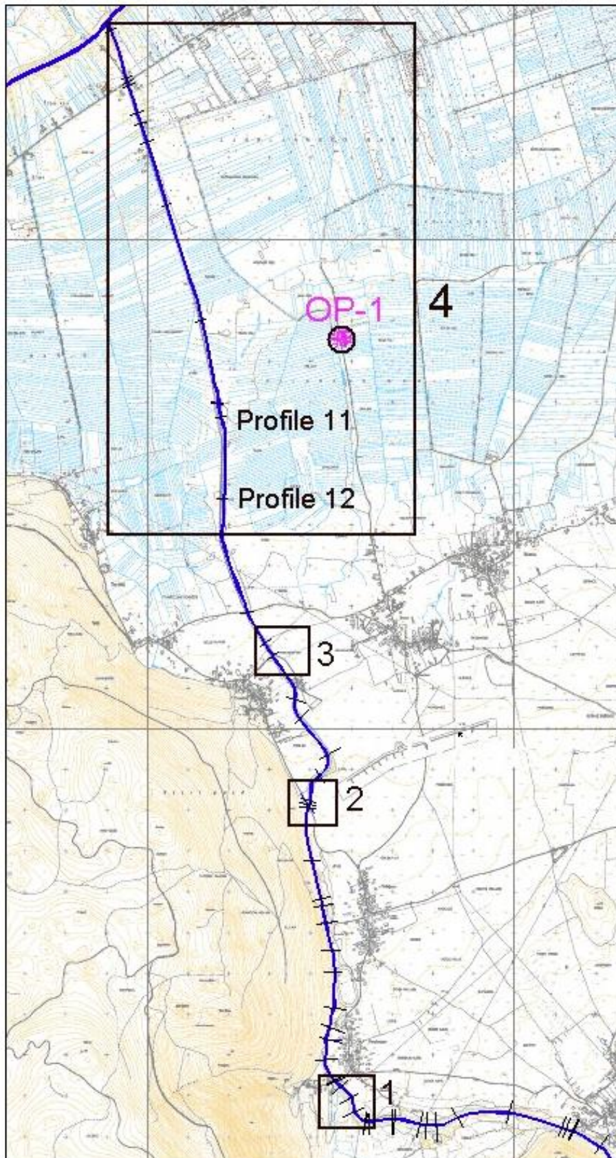
Slika 12: Lokacije preliivanja visoke vode (začetek poplav) na reki lški pri pretoku 97 \text{ m}^3/\text{s}
