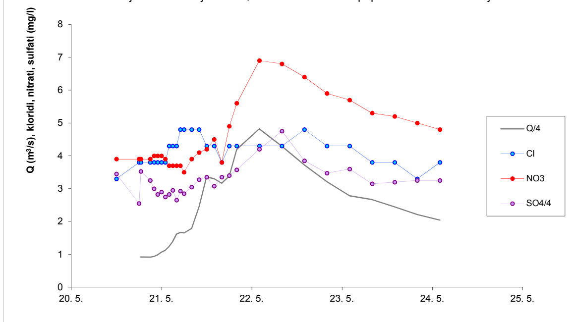
Nihanje koncentracij kloridov, nitratov in sulfatov v poplavnem valu Reke maja 1999.
